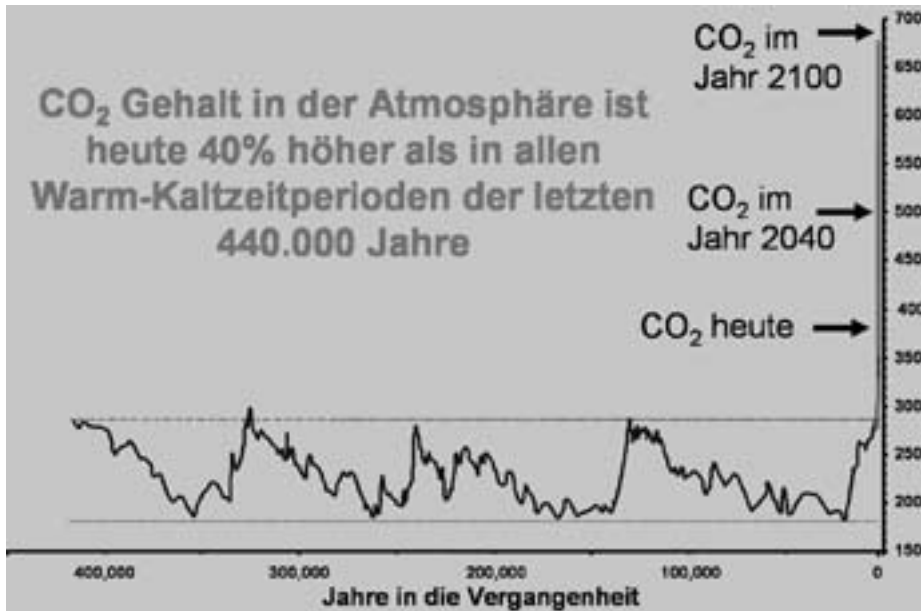
Entwicklung des CO 2 Gehalts in der Atmosphäre in den letzten 1/2 Million Jahren und heute. Der rapide Anstieg der letzten 100 Jahre ist verursacht durch die Verbrennung fossiler Energieträger und ist die Hauptursache der Ausbildung der Klimakatastrophe.
